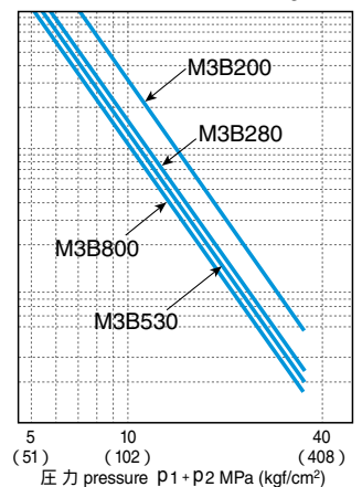
リヤ軸受寿命 / Rear bearing life
