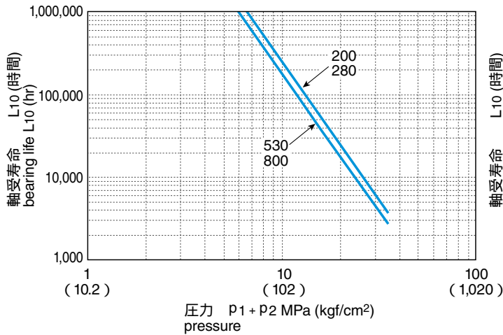
M3Xフロント軸受寿命 / Front bearing life
