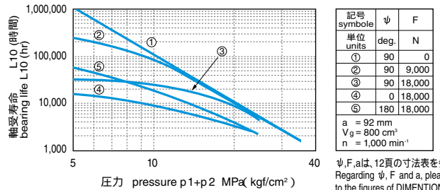
ラジアル荷重と軸受寿命 / Radial load and bearing life
