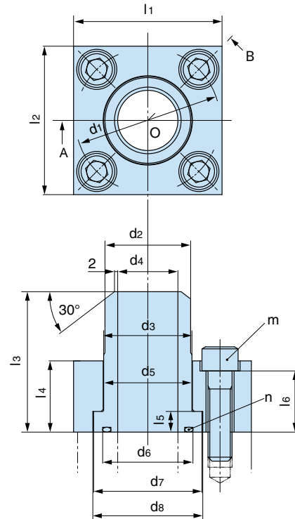
メインポート用フランジ/Flange for main ports
