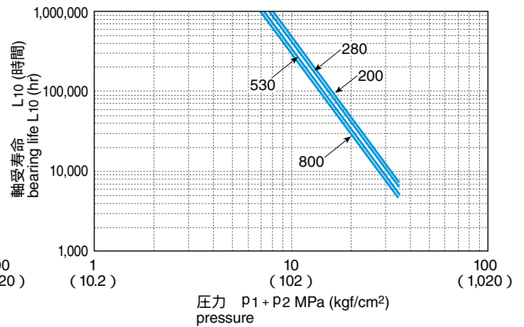
M3Xリヤ軸受寿命 / Rear bearing life
